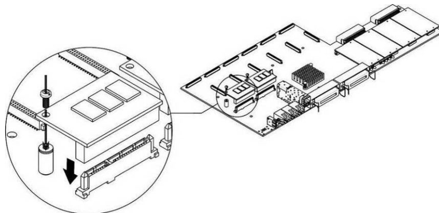
Рисунок 25 — Монтаж SSD-накопителя
