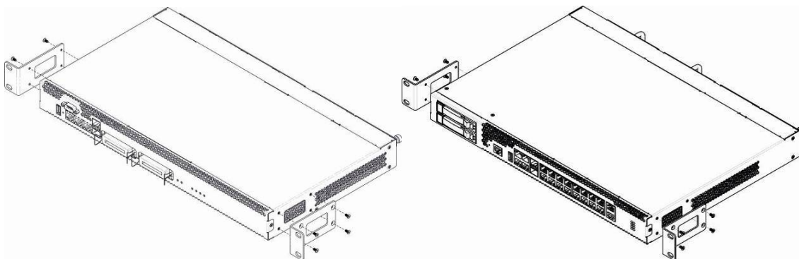
Рисунок 10 — Крепление кронштейнов для SBC-1000 (слева) и SBC-2000 (справа)
