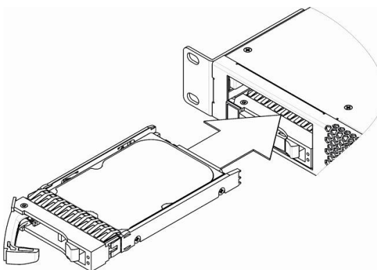
Рисунок 28 — Монтаж SATA-диска в корпус устройства
