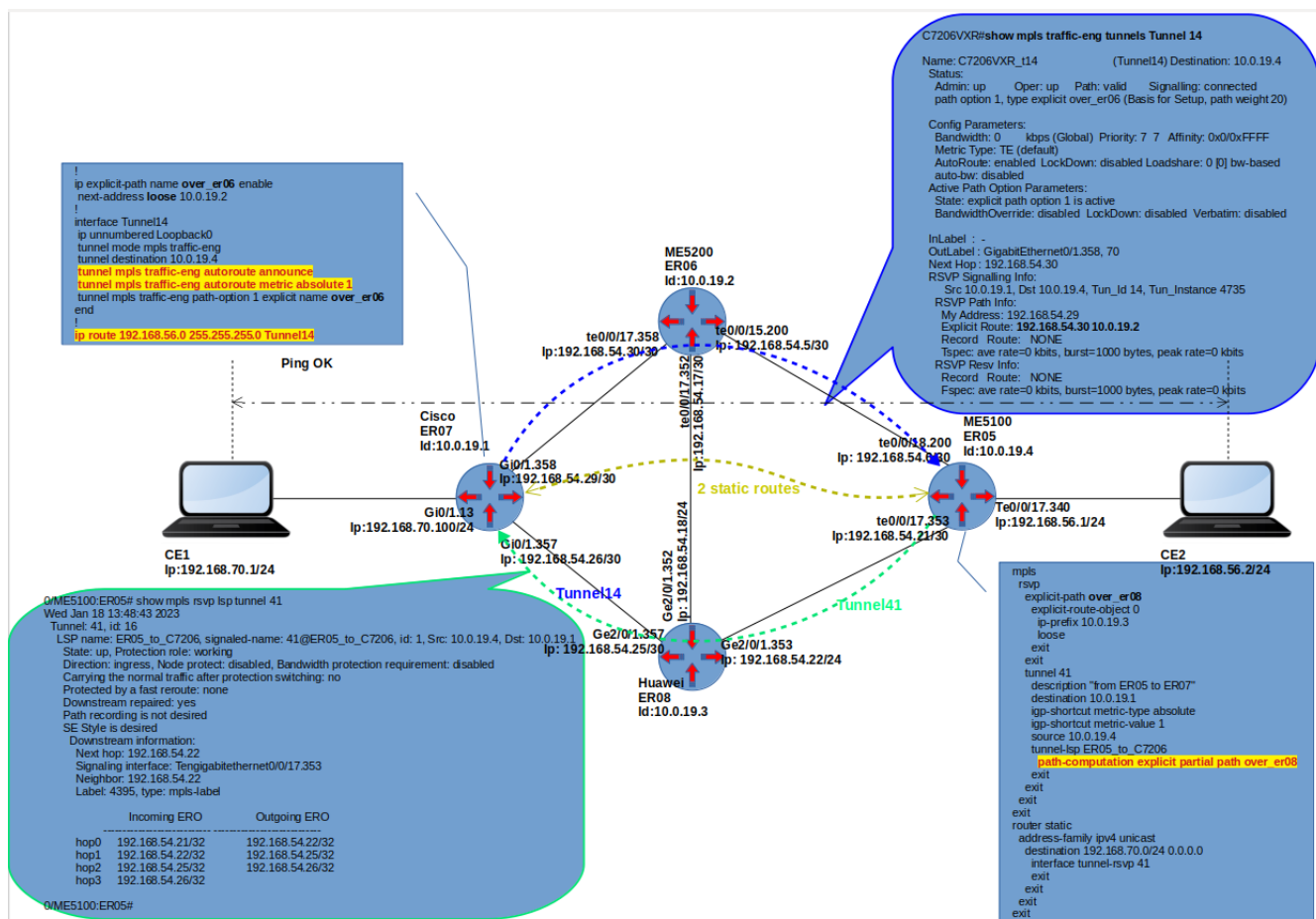
Figure 7. Передача трафика из GRT через TE-туннель с помощью статического маршрута
