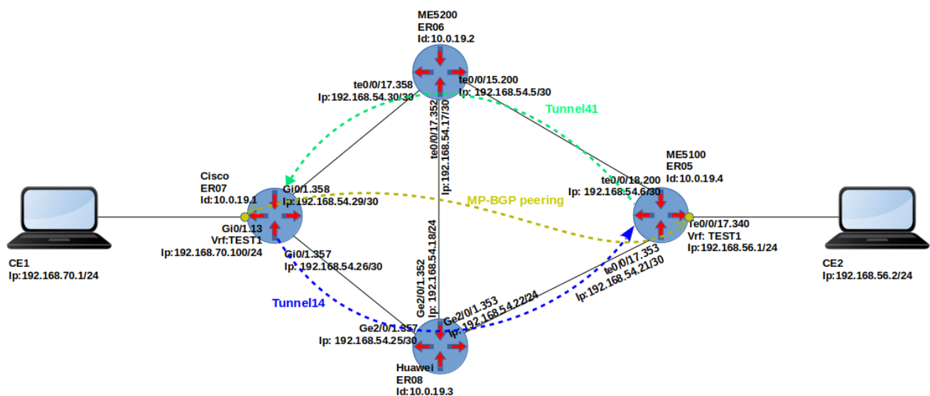
Figure 8. Передача сервисного трафика из VRF TEST1 через TE-туннель.
