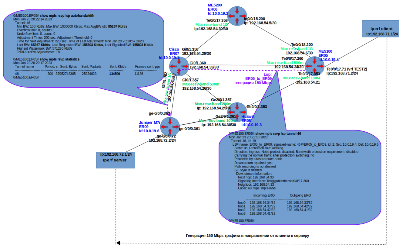
Figure 11. Как построится RSVP LSP 46@ER05_to_ER09 при генерации трафика 150 Mbps.
