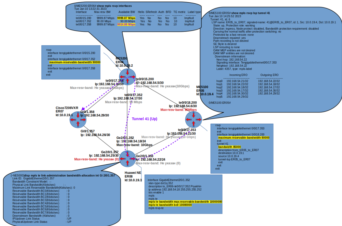
Figure 2. Конфигурация TE-туннеля с требованием резервирования полосы пропускания 85 Mbps.
