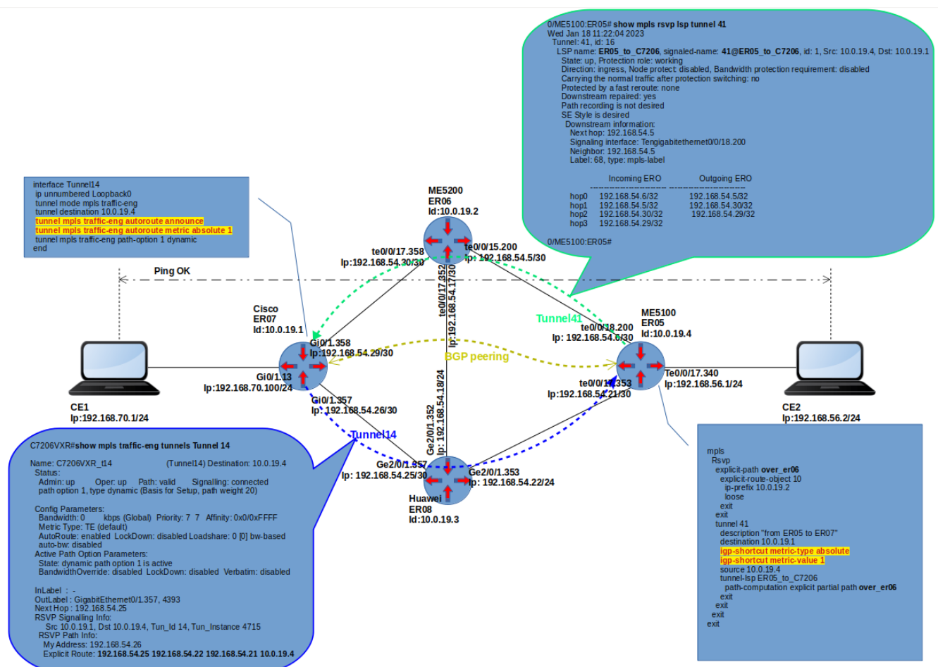
Figure 6. Передача трафика из GRT через TE-туннель
