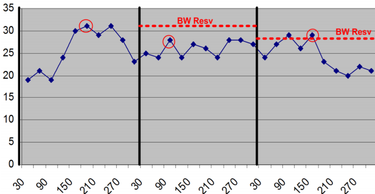
Figure 13. Пример профиля трафика и Adjust интервала в 300 секунд когда функционал работает хорошо.
