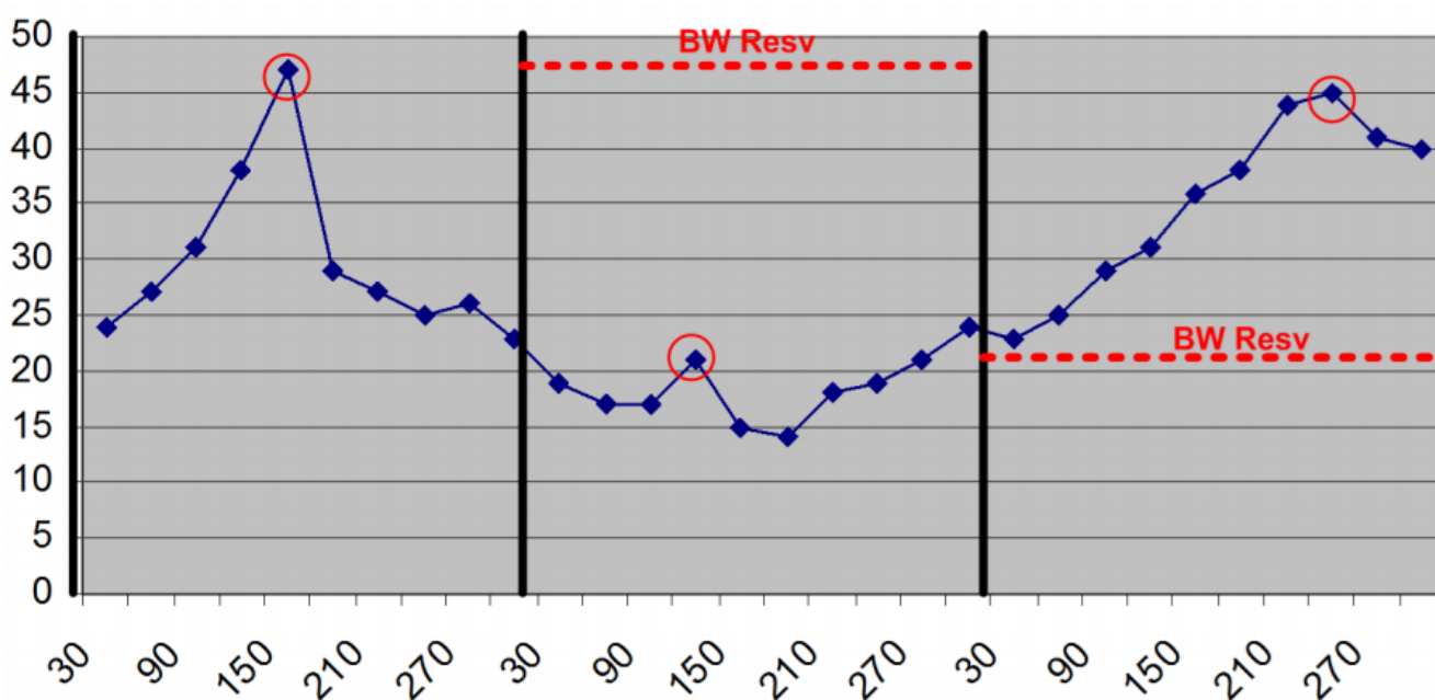
Figure 14. Пример профиля трафика и Adjust интервала в 300 секунд когда функционал работает плохо.
