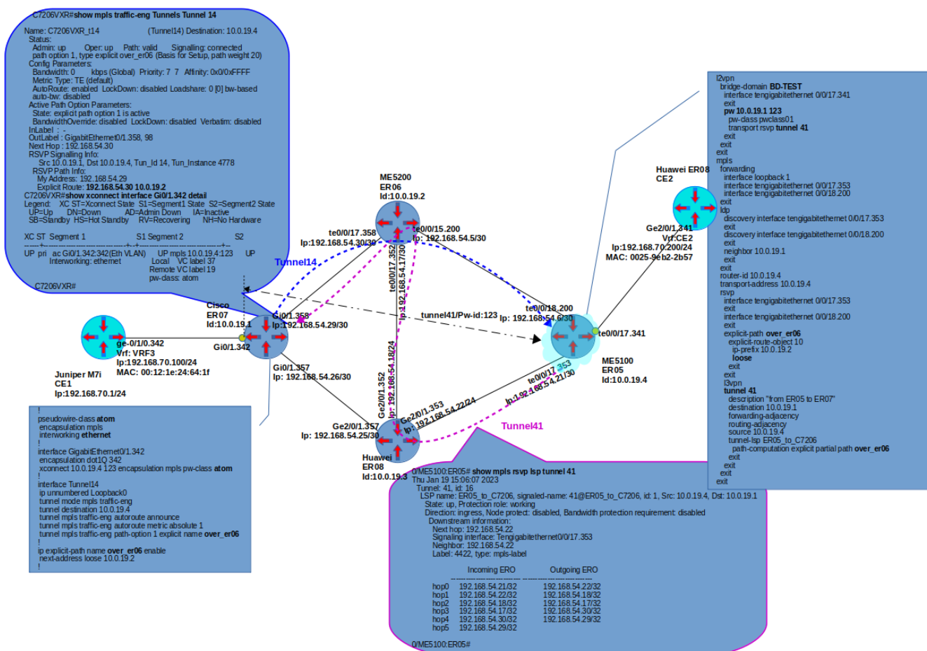
Figure 9. Передача сервисного трафика через L2VPN и TE-туннель.
