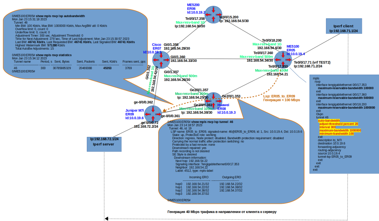
Figure 10. Начальное положение RSVP LSP 46@ER05_to_ER09 при генерации трафика до 100 Mbps.
