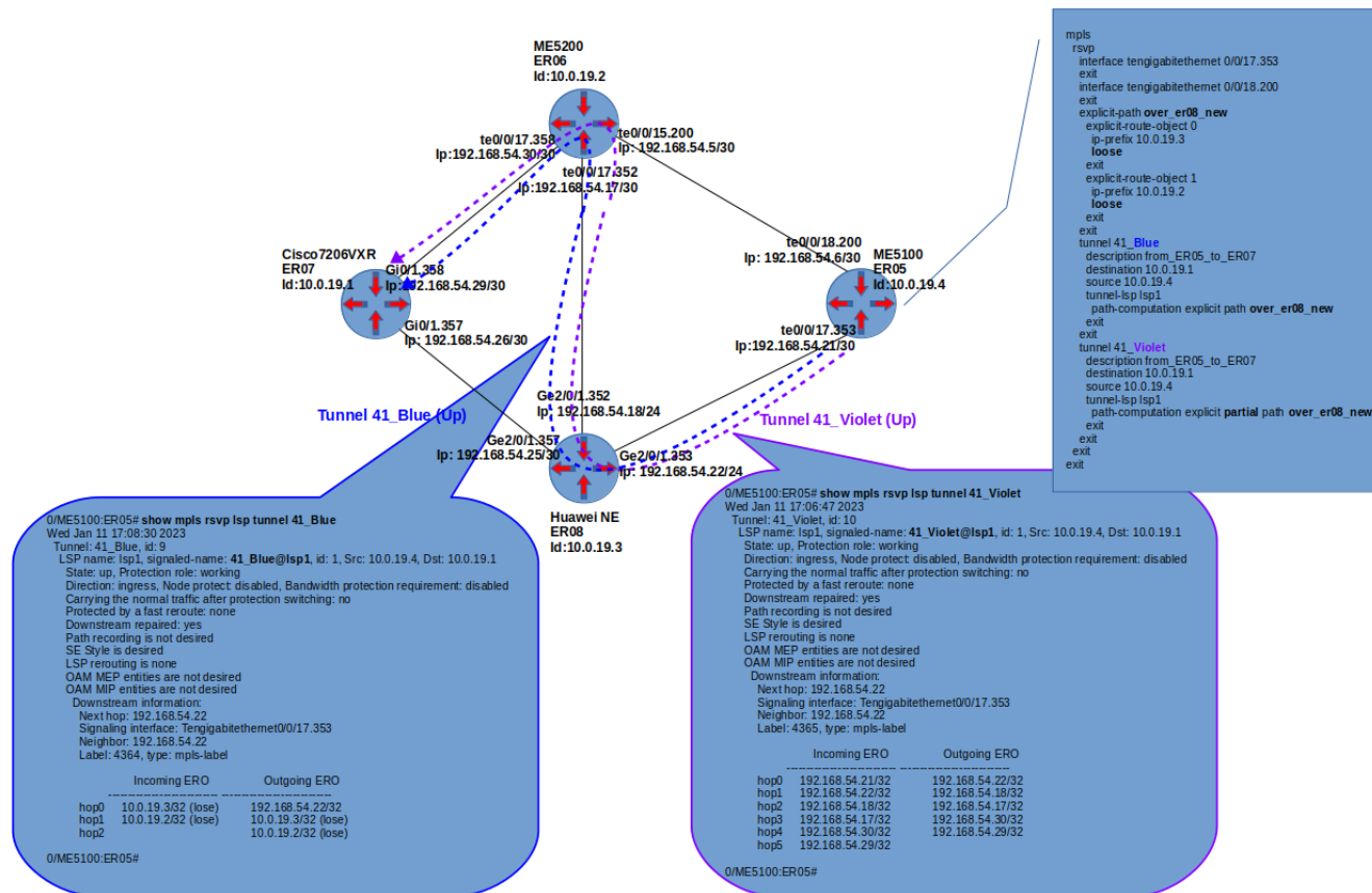
Figure 4. Конфигурация TE-туннелей с explicit path и опциями loose и partial.
