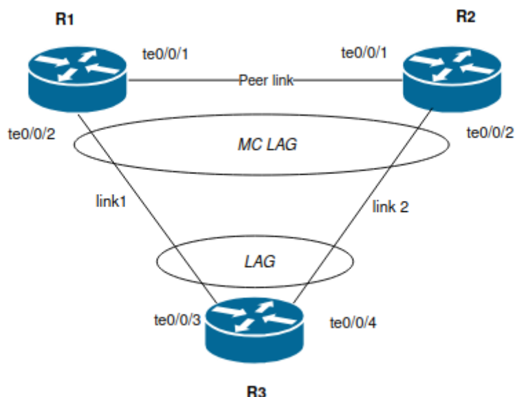
Figure 1. Схема организации MC-LAG
