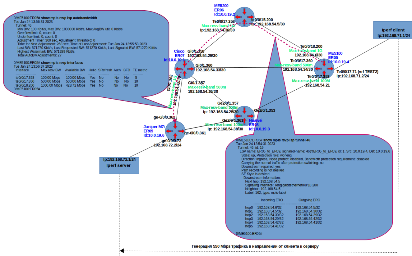
Figure 12. Как построятся RSVP LSP 46@ER05_to_ER09 при генерации трафика 550 Mbps.
