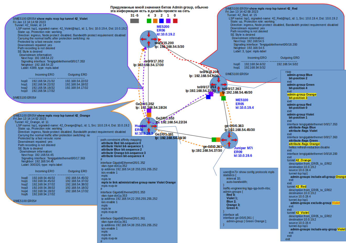
Figure 5. Конфигурация TE-туннеля с ограничением в виде Admin-Group.
