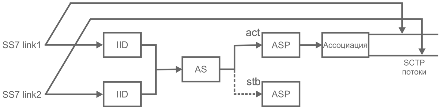
Рисунок 30 – Структурная схема процесса SGP
