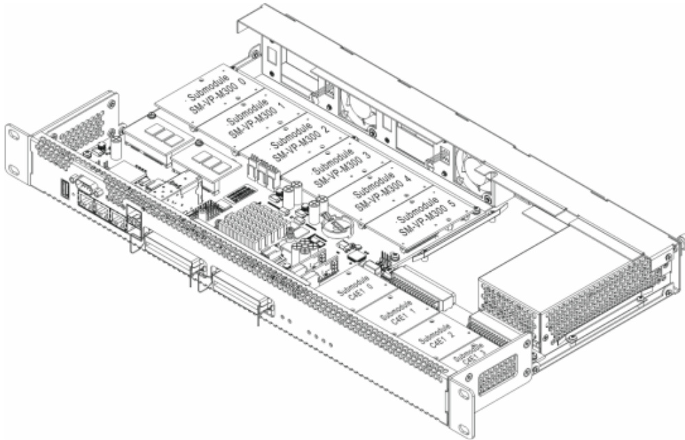
Рисунок 21 – Расположение субмодулей в SMG-1016M
