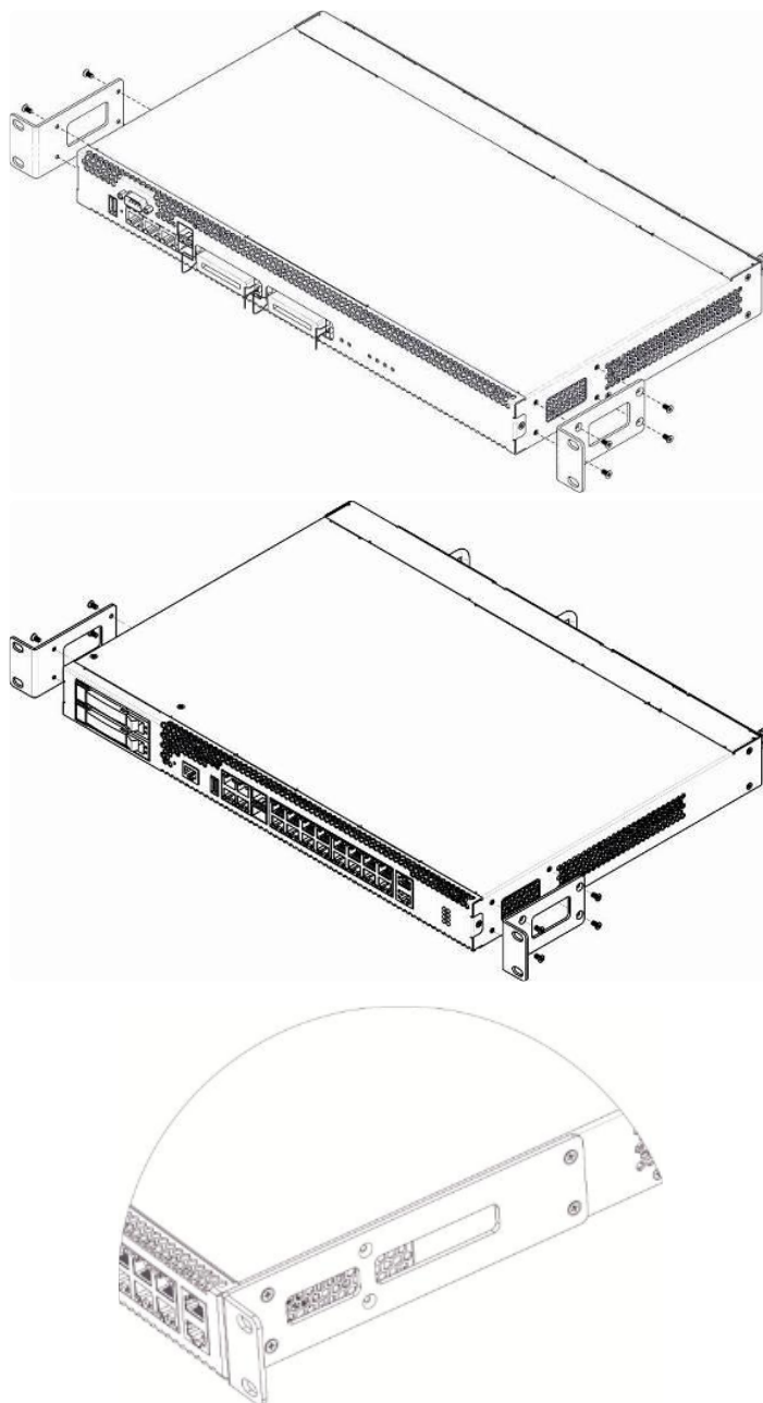
Рисунок 13 – Крепление кронштейнов для SMG-1016M (сверху слева), SMG-2016 (сверху справа) и SMG-3016 (внизу)
