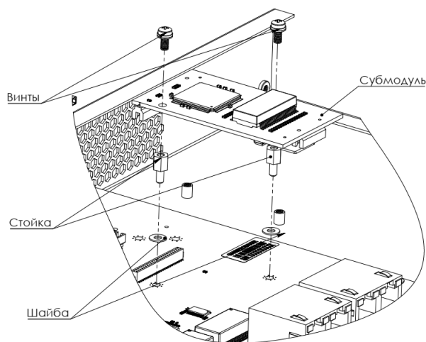
Рисунок 24 – Установка субмодуля на плату
