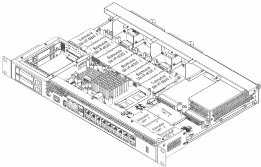
Рисунок 22 – Расположение субмодулей в SMG-2016
