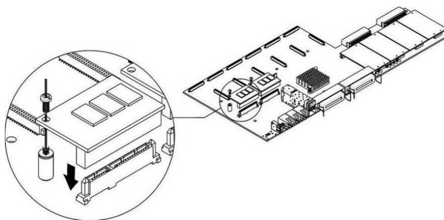
Рисунок 32 – Монтаж SSD-накопителя
