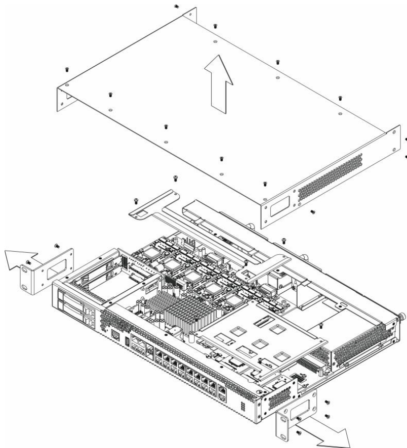
Рисунок 16 – Порядок вскрытия корпуса SMG-1016M
