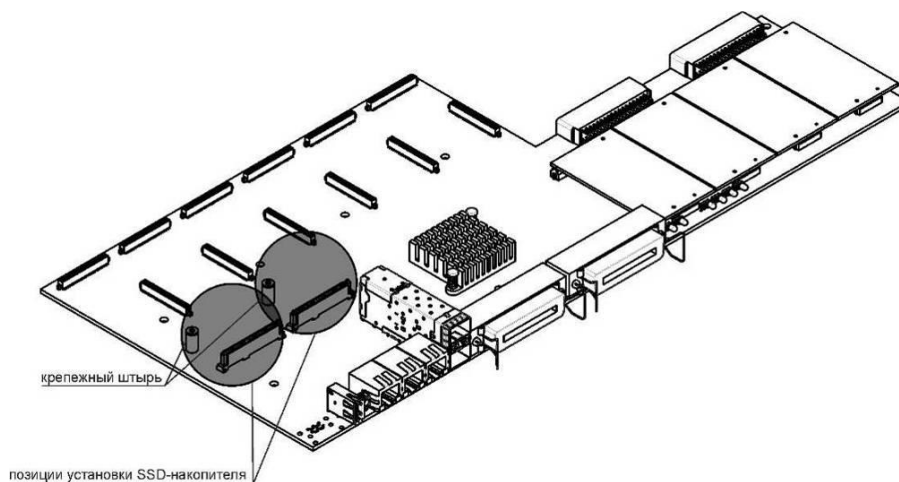
Рисунок 31 – Установка SSD-накопителя
