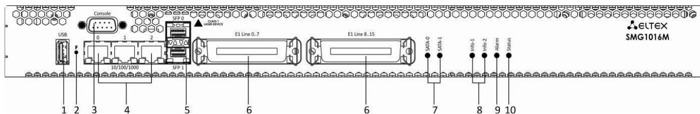
Рисунок 7 – Внешний вид передней панели SMG-1016M
