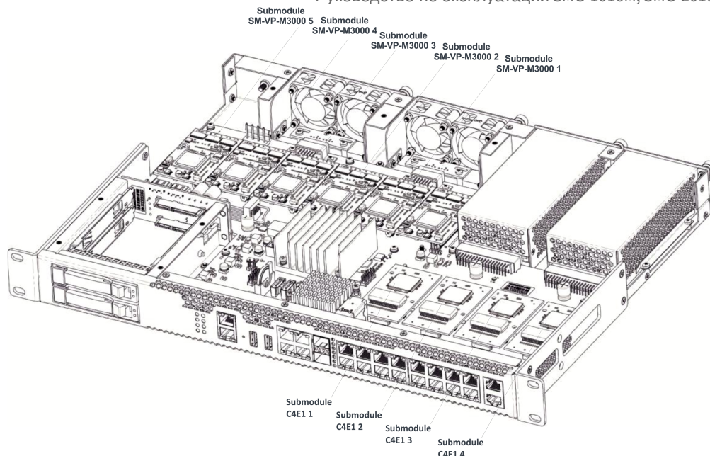
Рисунок 23 – Расположение субмодулей в SMG-3016
