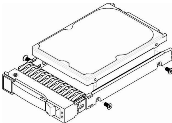
Рисунок 34 – Крепление SATA-диска в лоток направляющих салазок
