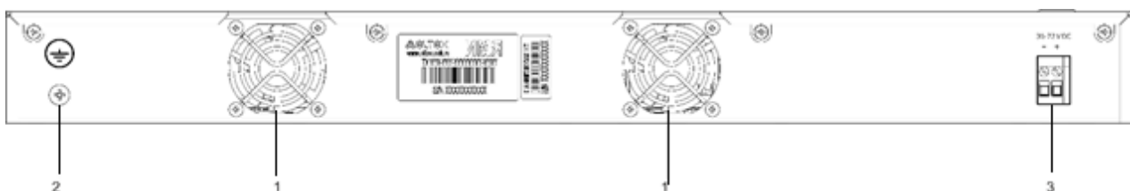
Рисунок 40 – Задняя панель MES2448 DC
