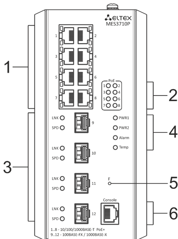
Рисунок 36 – Передняя панель MES3710P
