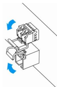
Рисунок 68 – Открытие защелки SFP-трансиверов
