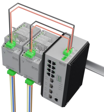
Рисунок 65 — Подключение питания коммутатора от двух блоков питания DRS-270-56
