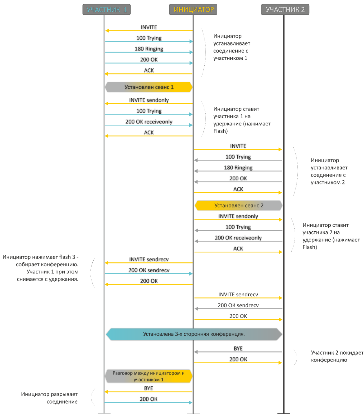
Рисунок 19 – Алгоритм выполнения услуги «Трёхсторонняя конференция» («3-way conference») локально на устройстве по протоколу SIP
