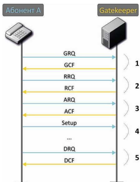
Рисунок 26 – Алгоритм вызова через гейткипер
