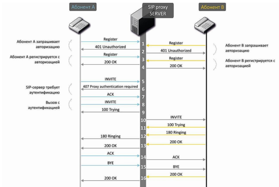
Рисунок 23 – Алгоритм вызова с участием SIP проху-сервера
