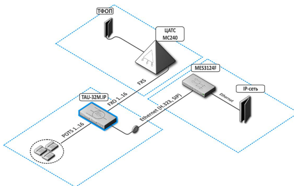
Рисунок 5 – Схема использования TAU-32M.IP в качестве FXS+FXO
