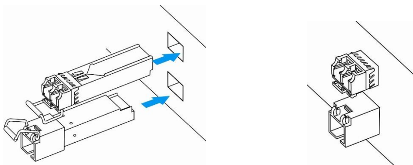
Рисунок 15 – Установка SFP-трансиверов
