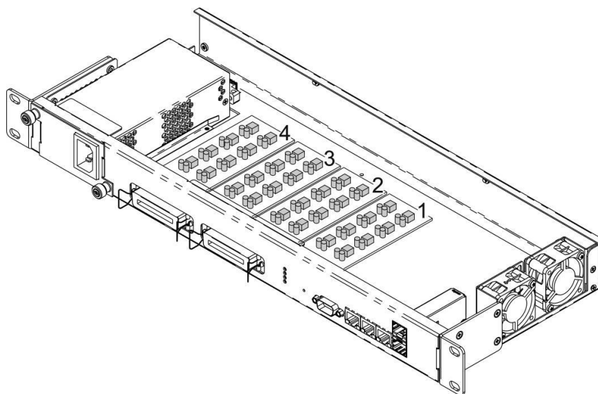
Рисунок 14 – Расположение субмодулей в TAU-32M.IP
