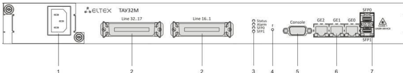
Рисунок 7 – Внешний вид передней панели TAU-32M.IP
