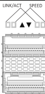
Рисунок 84 – Внешний вид разъема QSFP+ и QSFP28 для MES5300-48, MES5305-48, MES5310-48, MES5400-xx, MES5410-48
