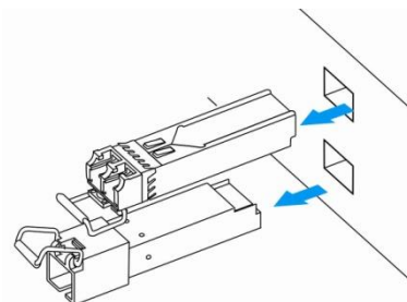
Рисунок 52 — Извлечение SFP-трансиверов
