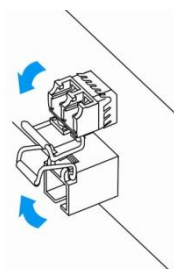
Рисунок 51 — Открытие защелки SFP-трансиверов
