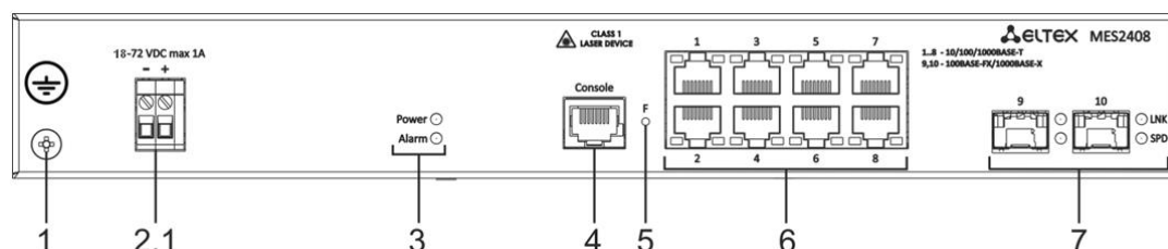
Рисунок 4 – Передняя панель MES2408 DC
