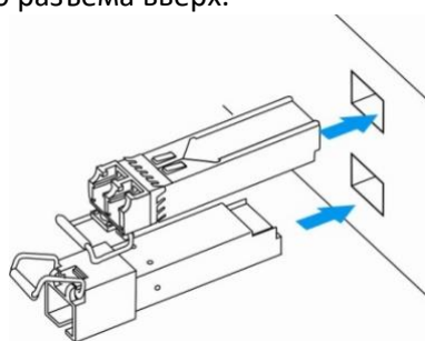
Рисунок 66 – Установка SFP-трансиверов
