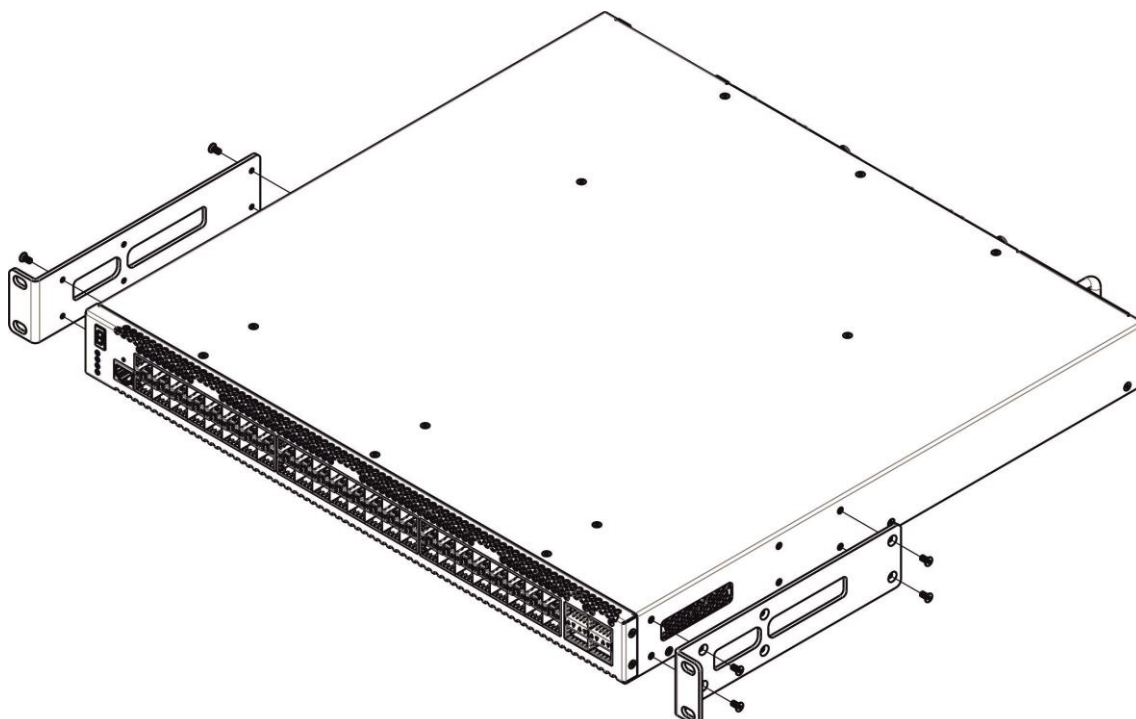
Рисунок 11 – Крепление кронштейнов
