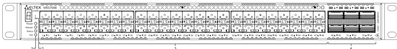
Рисунок 5 – Передняя панель MES7048
