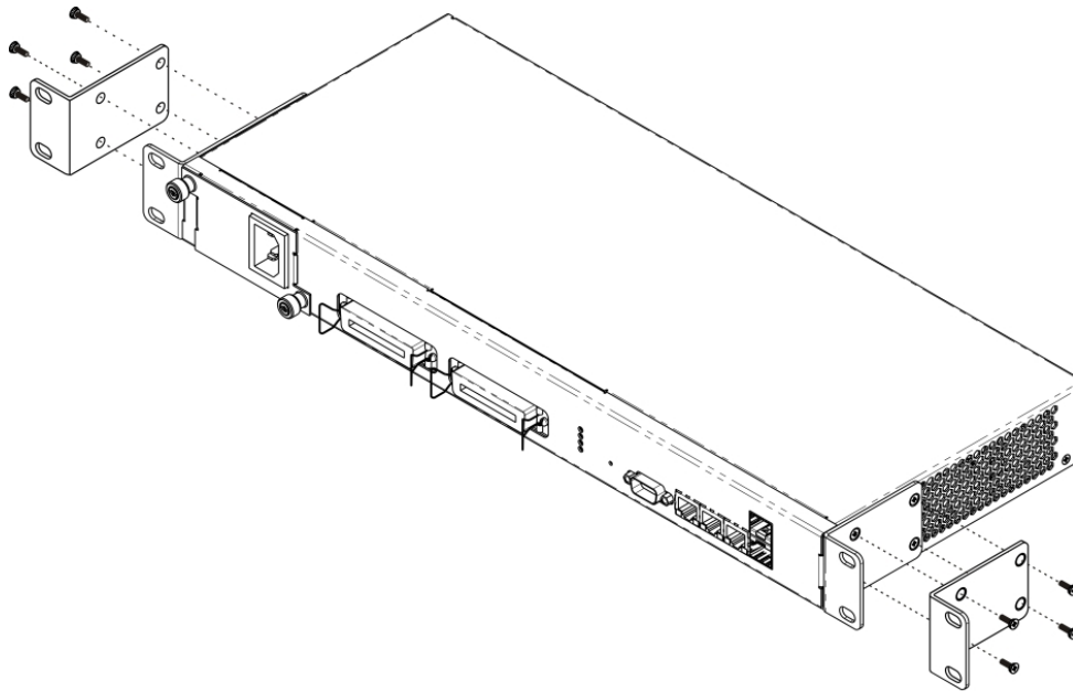
Рисунок 11 – Крепление кронштейнов
